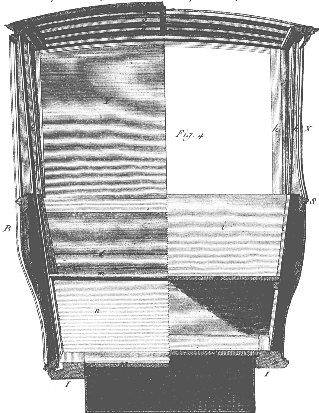
Coupe sur la ligne a. b A Coupe sur la ligne c. d.
