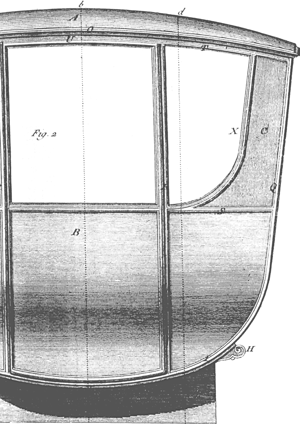
Elevation d'une Berline
